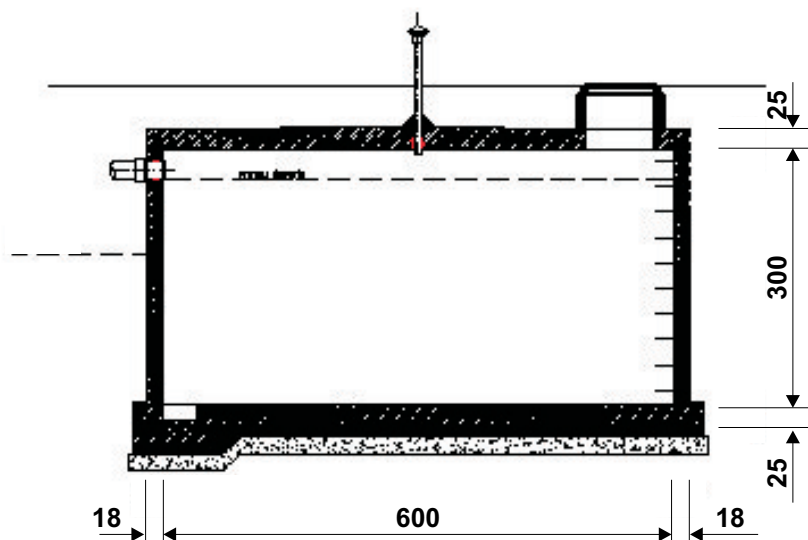
PRZEKRÓJ
