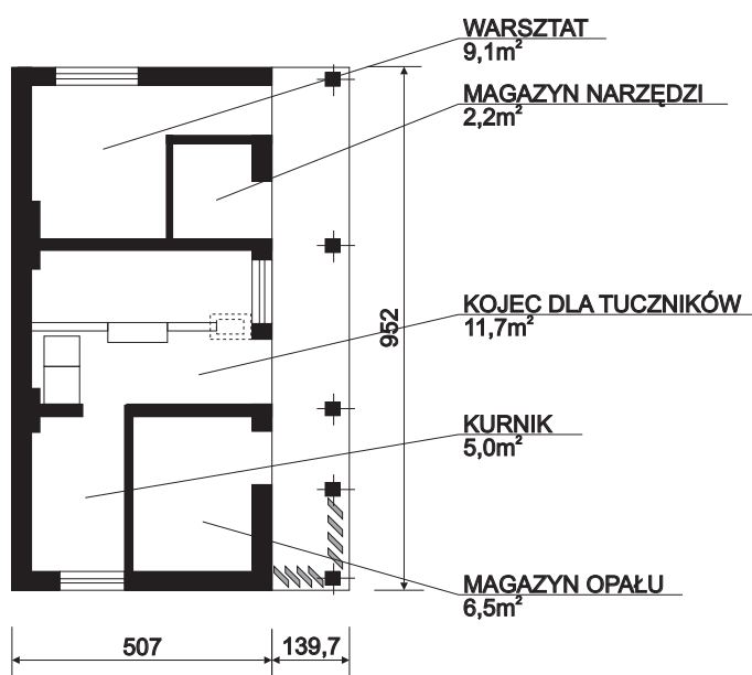
PRZYZIEMIE
