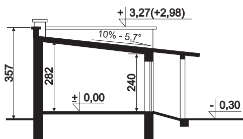
PRZEKRÓJ
