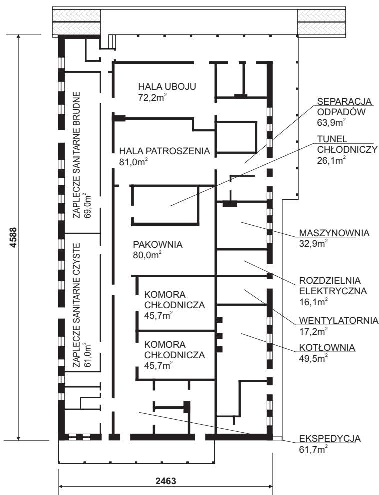
RZUT PRZYZIEMIA
