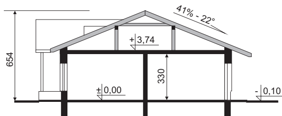
PRZEKRÓJ
