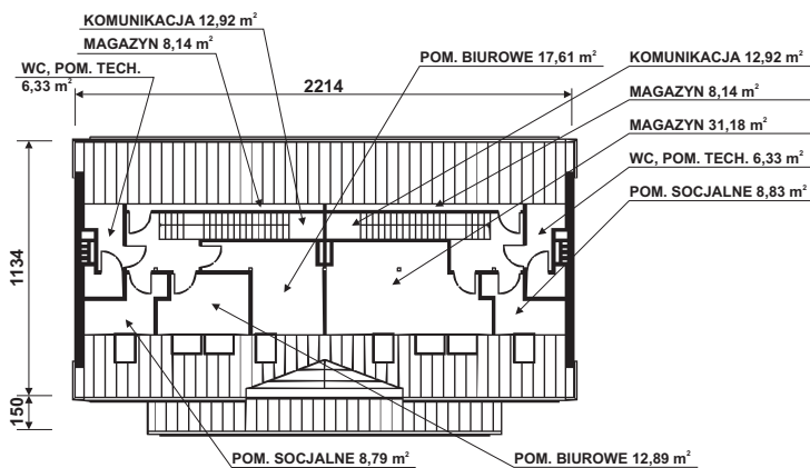
RZUT PODDASZA
