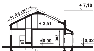
PRZEKRÓJ
