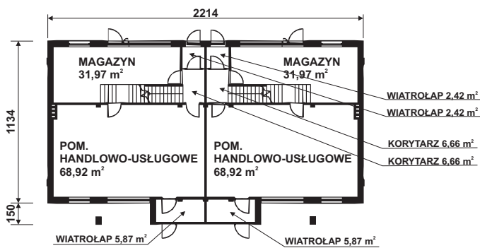
RZUT PARTERU
