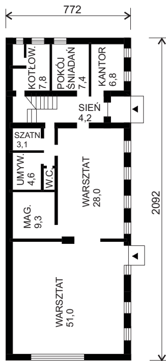
PRZYZIEMIE
