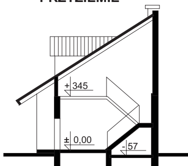
PRZEKRÓJ
