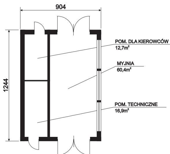
PRZYZIEMIE
