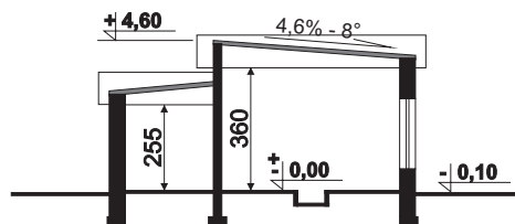
PRZEKRÓJ
