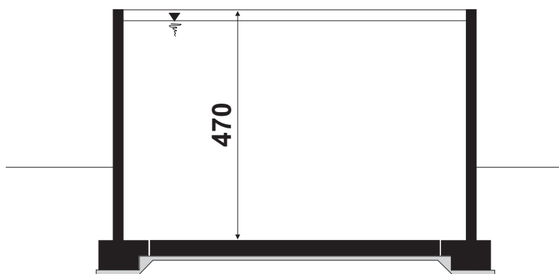
PRZEKRÓJ
