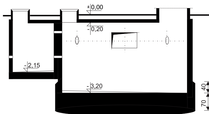
PRZEKRÓJ
