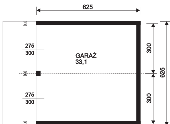
RZUT PRZYZIEMIA
