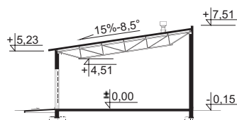
PRZEKRÓJ
