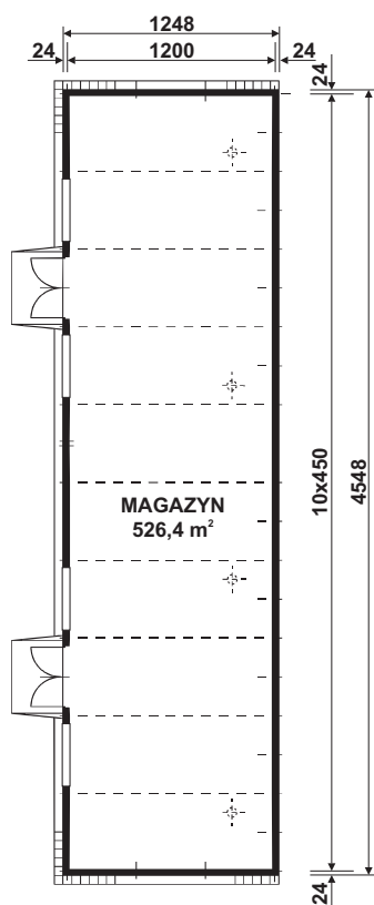
RZUT PRZYZIEMIA
