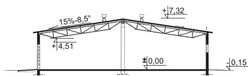
PRZEKRÓJ
