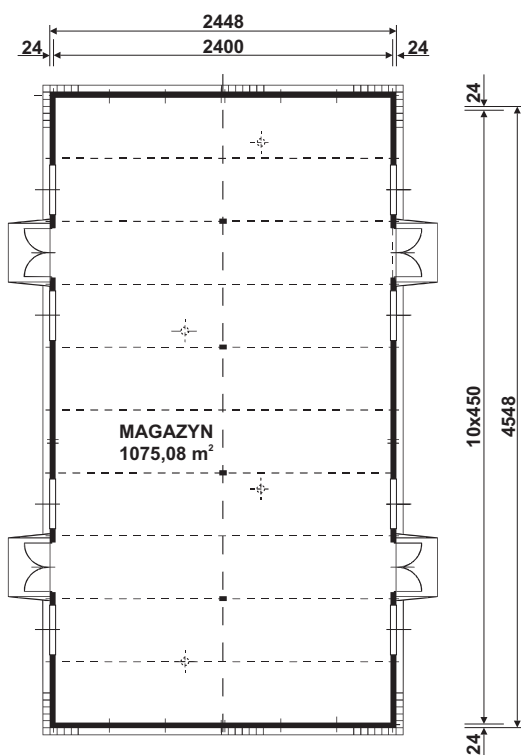
RZUT PRZYZIEMIA
