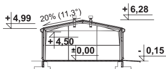
PRZEKRÓJ
