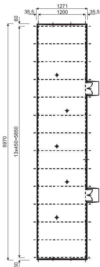
PRZYZIEMIE
