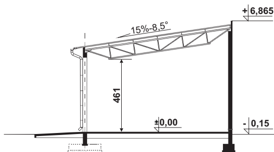
PRZEKRÓJ
