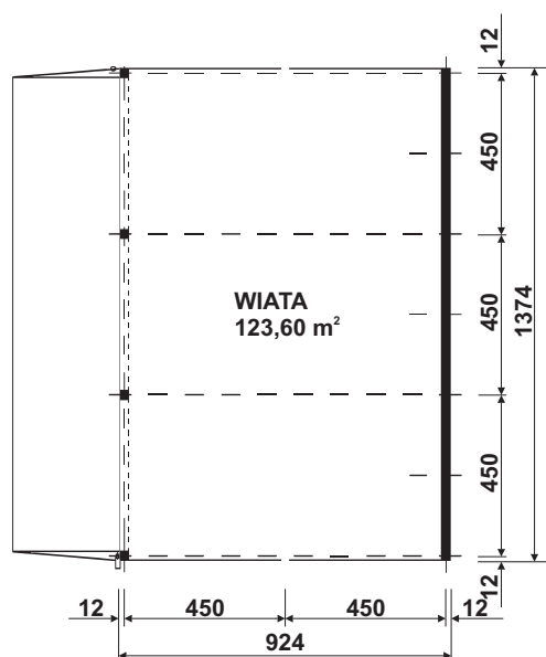
RZUT PRZYZIEMIA
