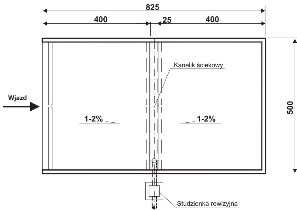
RZUT
