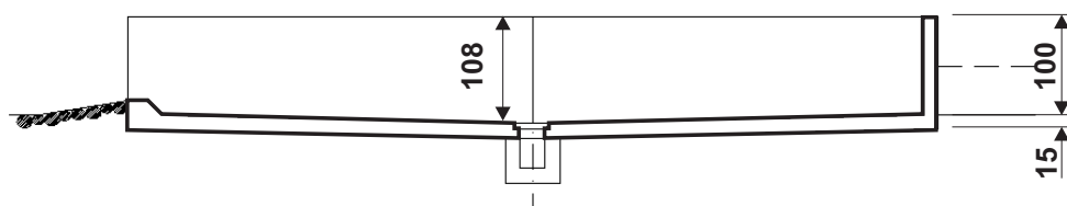
PRZEKRÓJ
